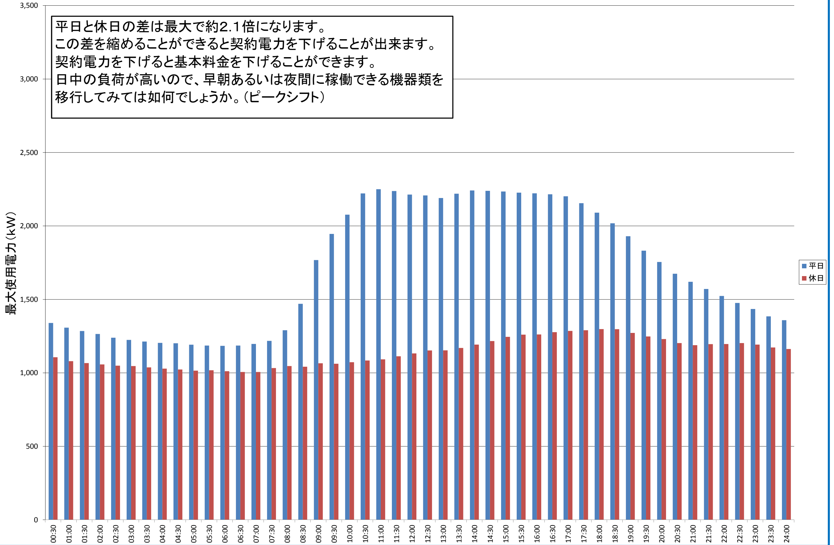
黒髪南キャンパス 1月の時間帯別最大使用電力平均値
