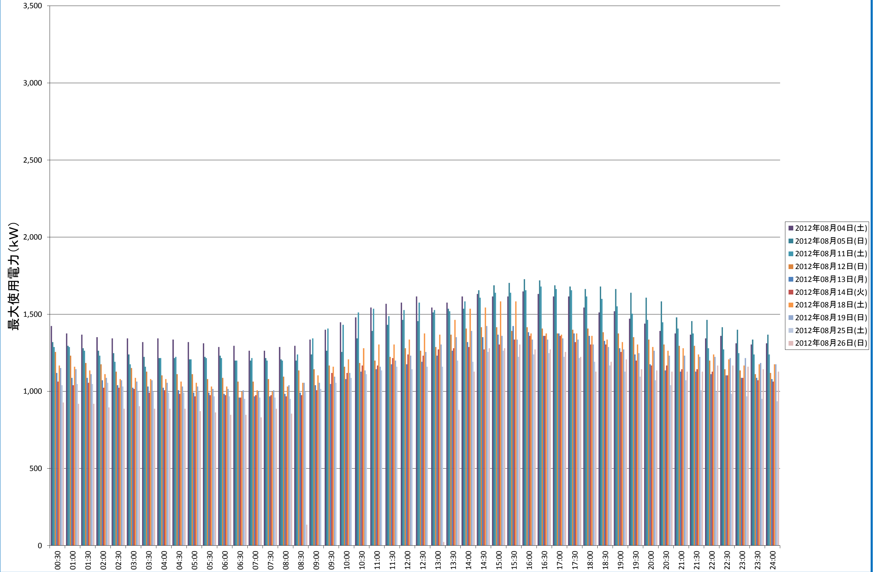
黒髪南キャンパス 8月の時間帯別最大使用電力(土日祝)
