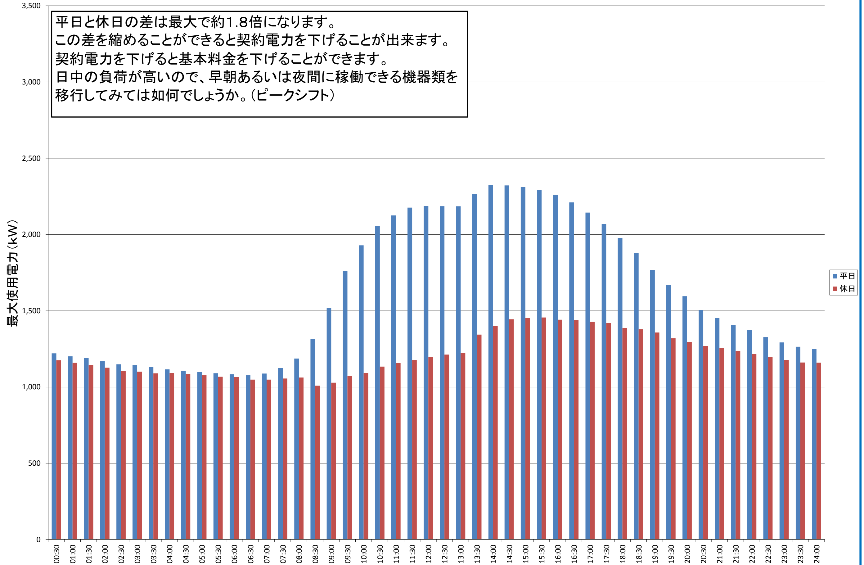
黒髪南キャンパス 8月の時間帯別最大使用電力平均値
